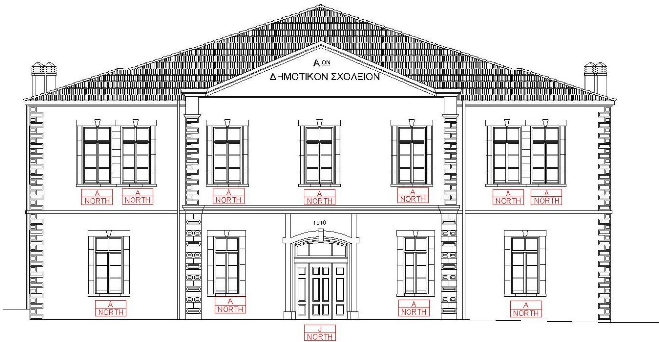
Σκαρίφημα 2: Κουφώματα στην πλευρά NORTH
