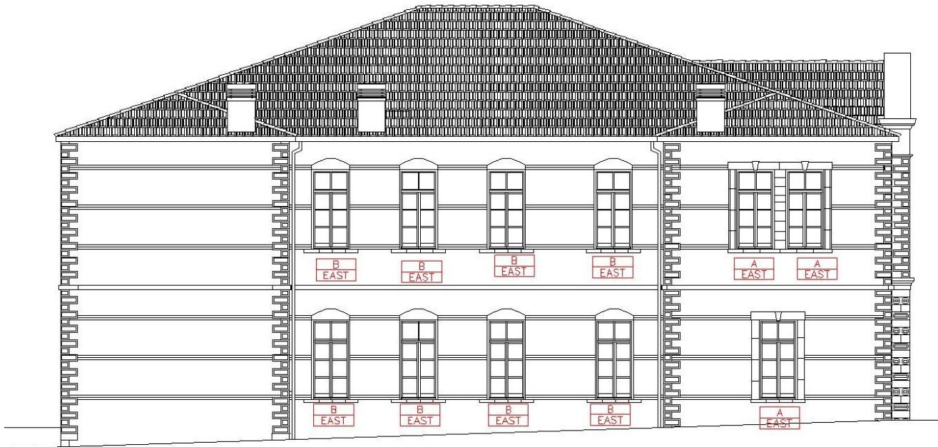
Σκαρίφημα 1: Κουφώματα στην πλευρά EAST
